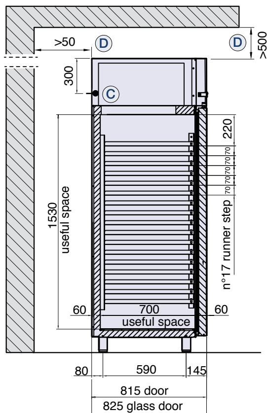
A-A
